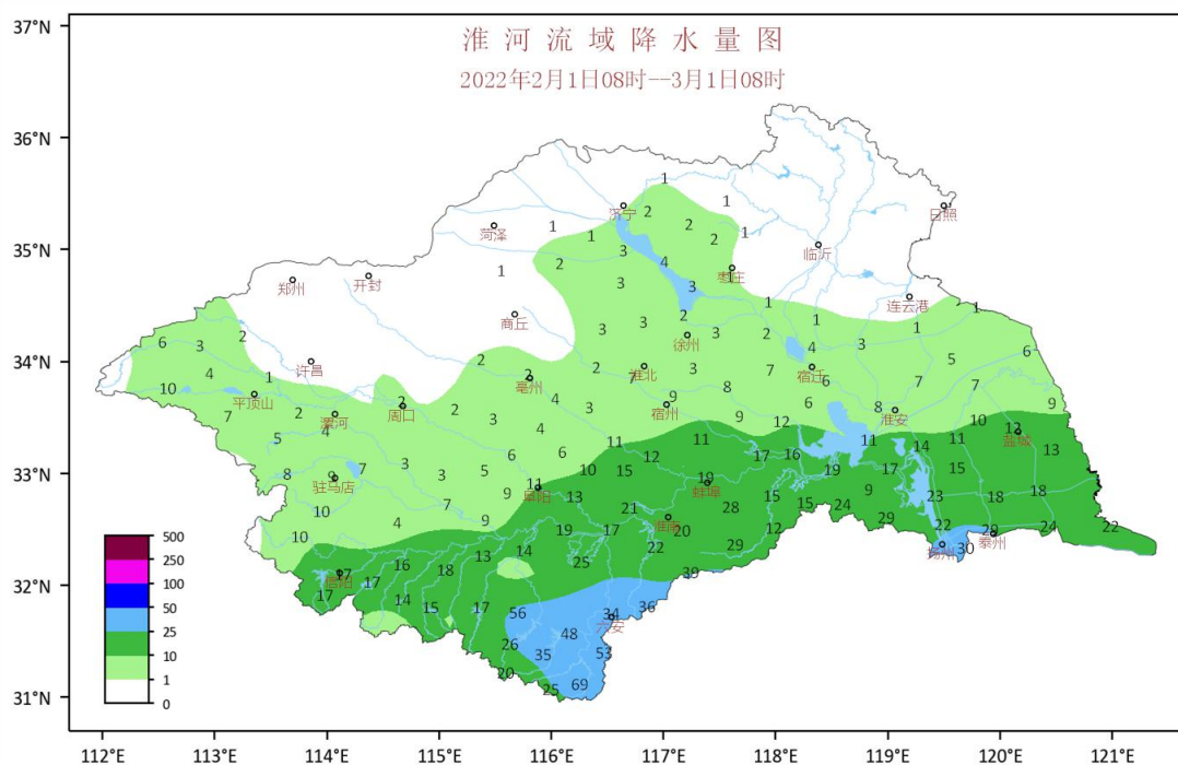
图 1 2022 年 2 月淮河流域降水量分布图
