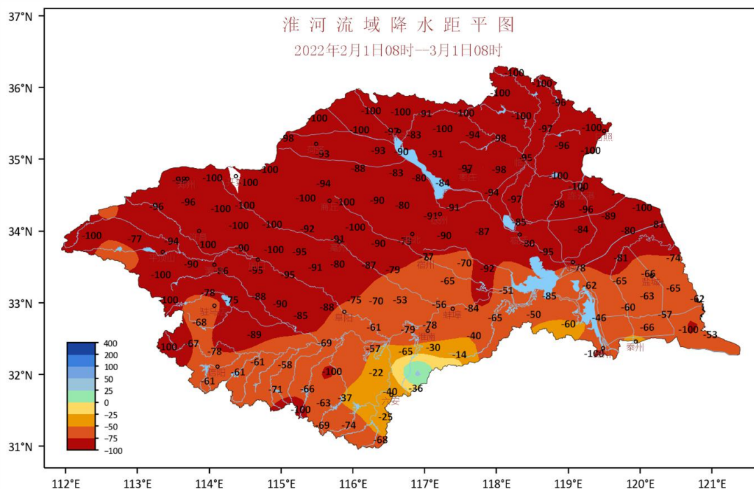
图 2 2022 年 2 月淮河流域降水量距平图
