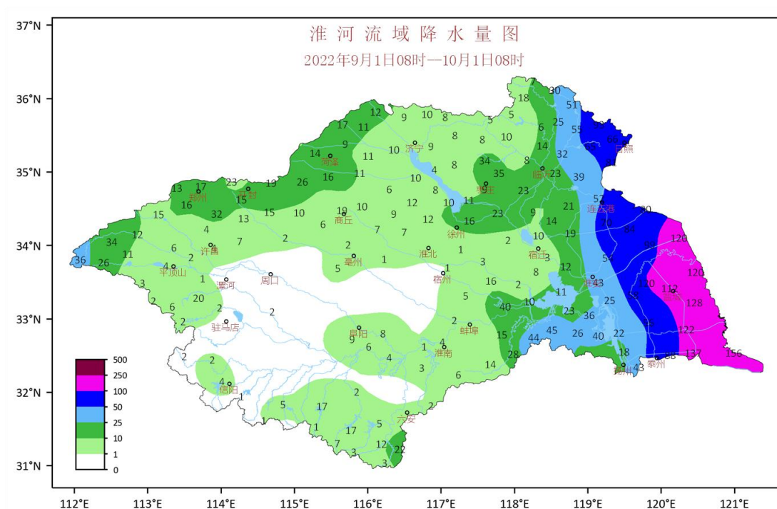
图 1 2022 年 9 月淮河流域降水量分布图
