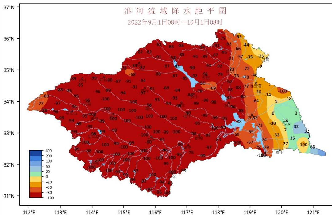
图 2 2022 年 9 月淮河流域降水量距平图
