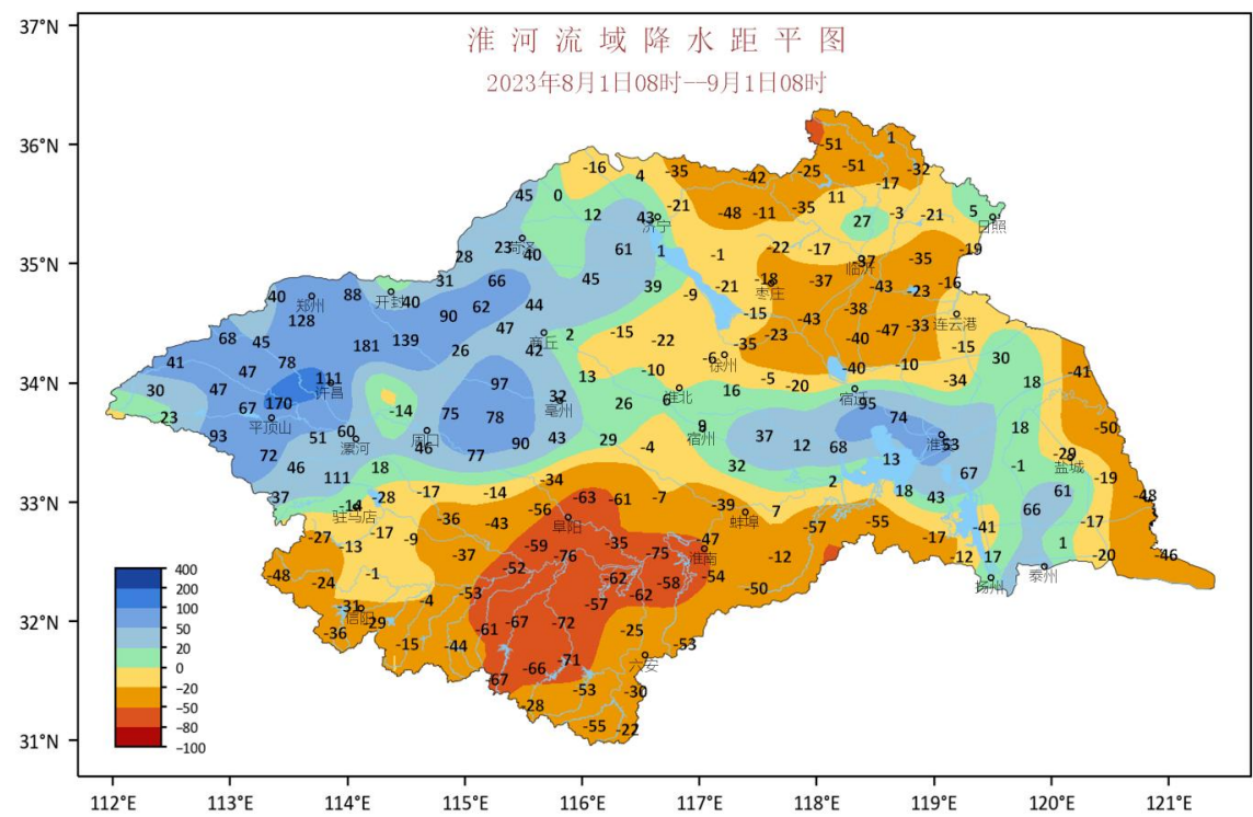
图 2 2023 年 8 月淮河流域降水量距平图
