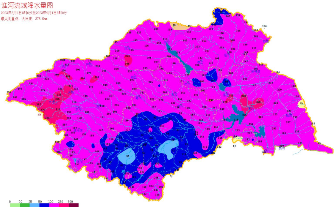
图 1 2023 年 8 月淮河流域降水量分布图
